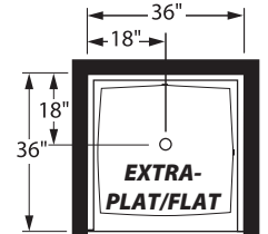
seuil/threshold 2" EXTRA-PLAT/FLAT 36" X 36"
