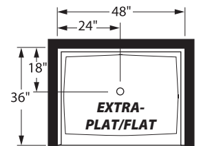
seuil/threshold 2" EXTRA-PLAT/FLAT 48" X 36"
