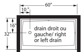
seuil/threshold 4 1/2" drain droit ou gauche/ right or left drain 60" X 32"
